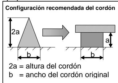
Figura 1: configuración recomendada de la cama de adhesivo.
